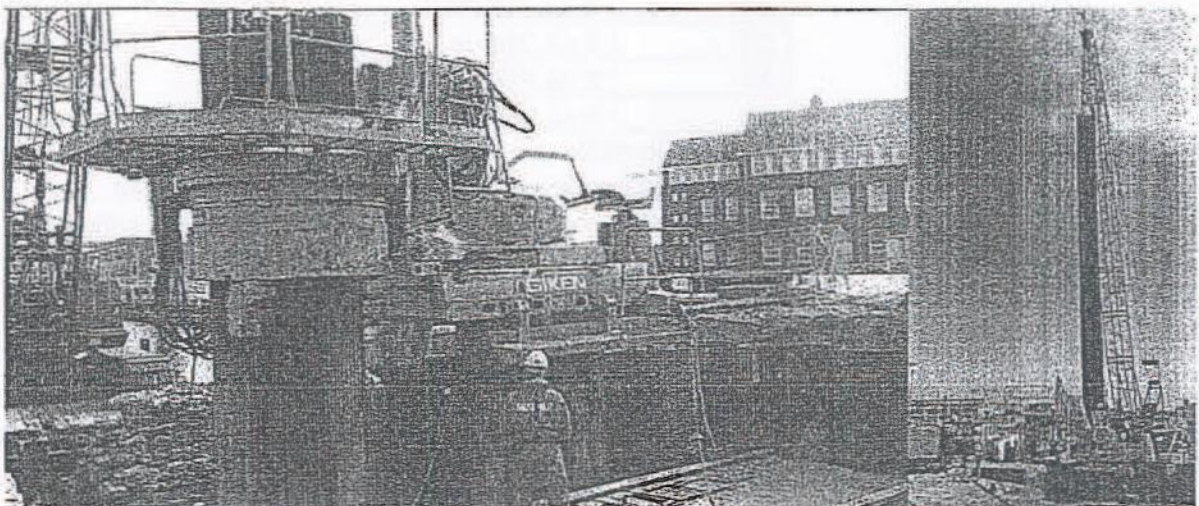
Inzet Giken Silent Piler drukmachine met kraanponton voor aanvoer van de damwand
