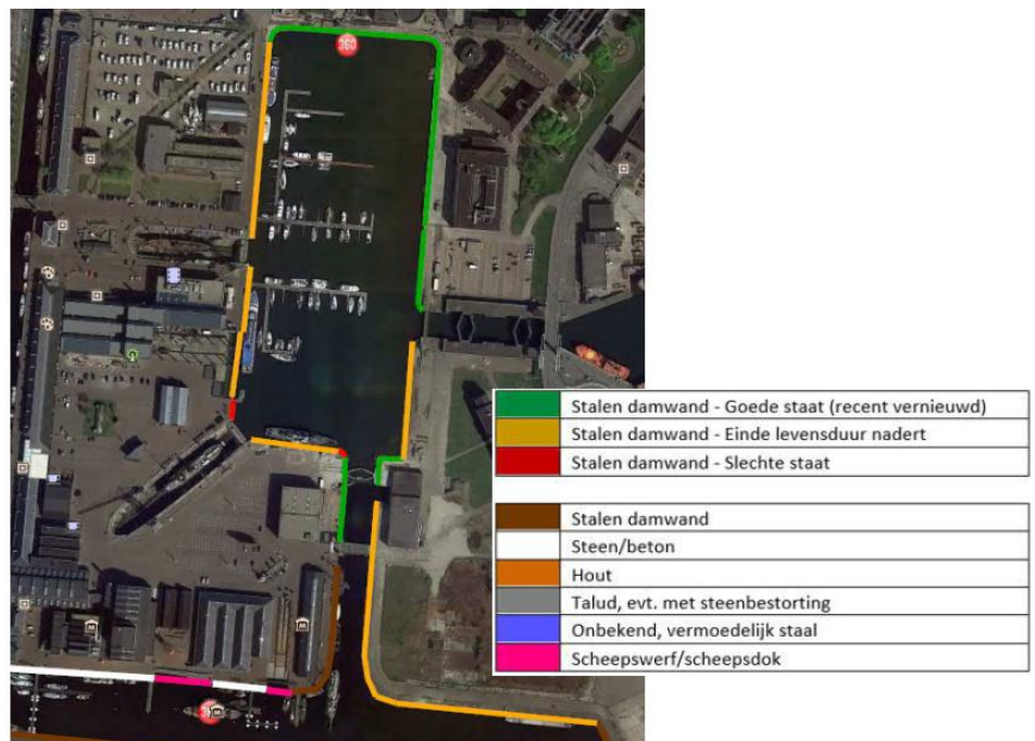
Figuur 11. Staat van de kades. Bron: Onderzoek KVSS 2019.
